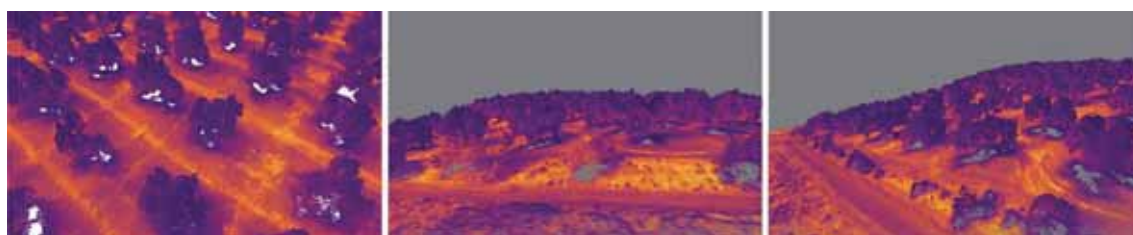
Figura 6: Caracterización termográfica de una plantación de olivar ubicada en la localidad de Mancha Real. Estos resultados son visualizados con el visor de GEU.
