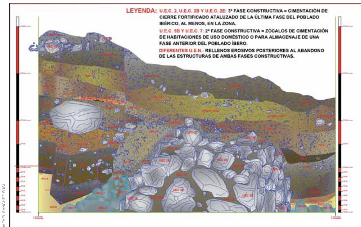
Fig. 16. Dibujo procesado en Autocad de la proyección del perfil estratigráfico NE. del sondeo abierto en el centro del carril de la c/ Cerro Alto de Martos con dos de las tres fases constructivas-estratigráficas diferentes de un asentamiento de época íbera plena.
