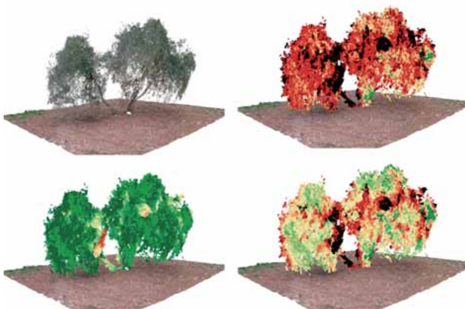
Figura 5: Caracterización de olivos aislados considerando distintos índices de vegetación (RVI, NDRE y NDVI), que son calculados a partir de los valores de reflectancia observados.
